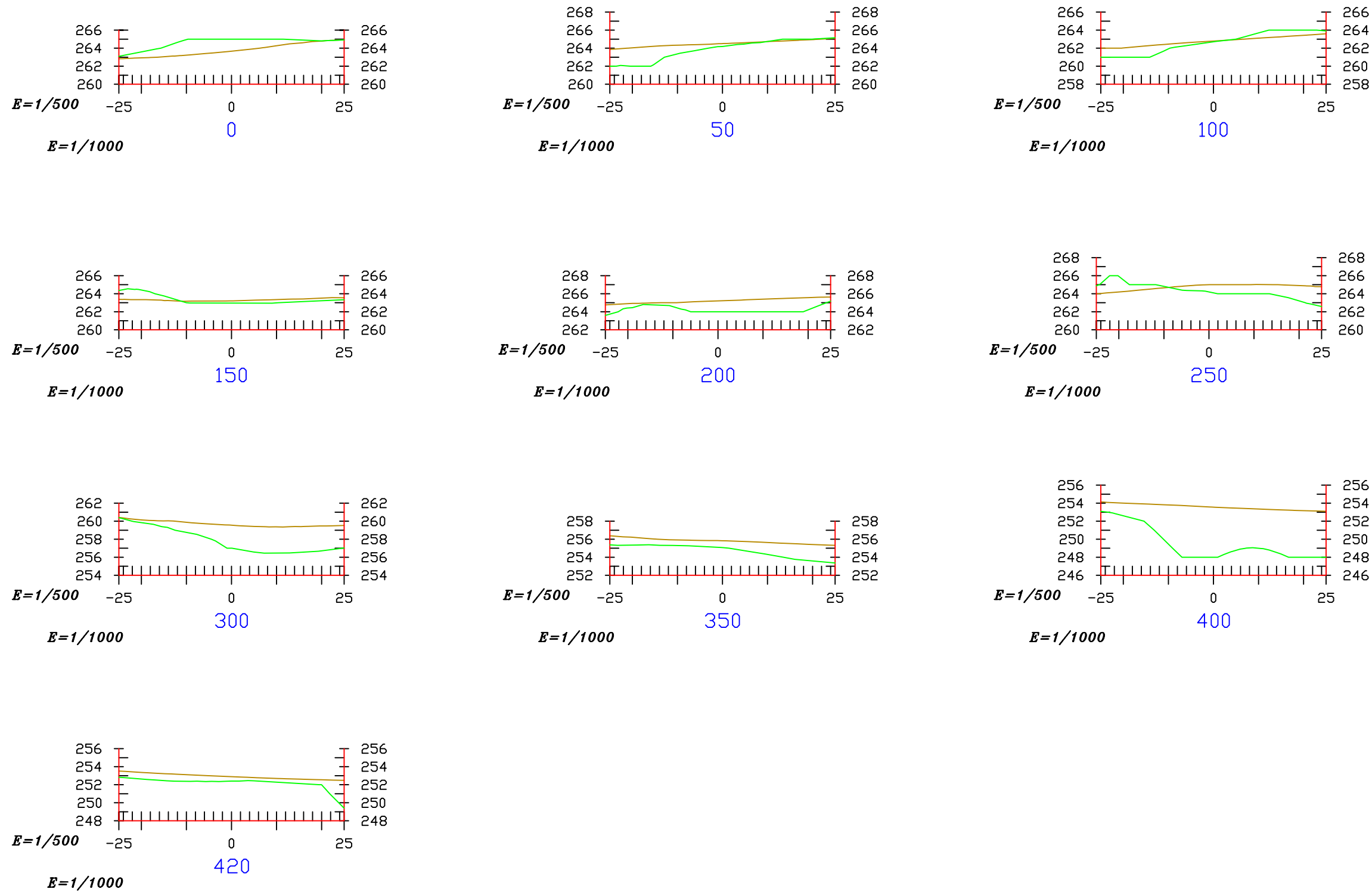
Perfiles Transversales (Secciones cada 50 m)
