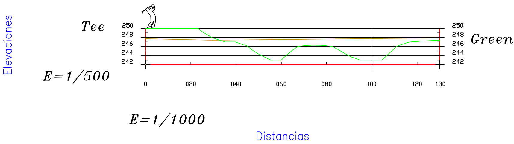
Perfil Longitudinal Hoyo 11
