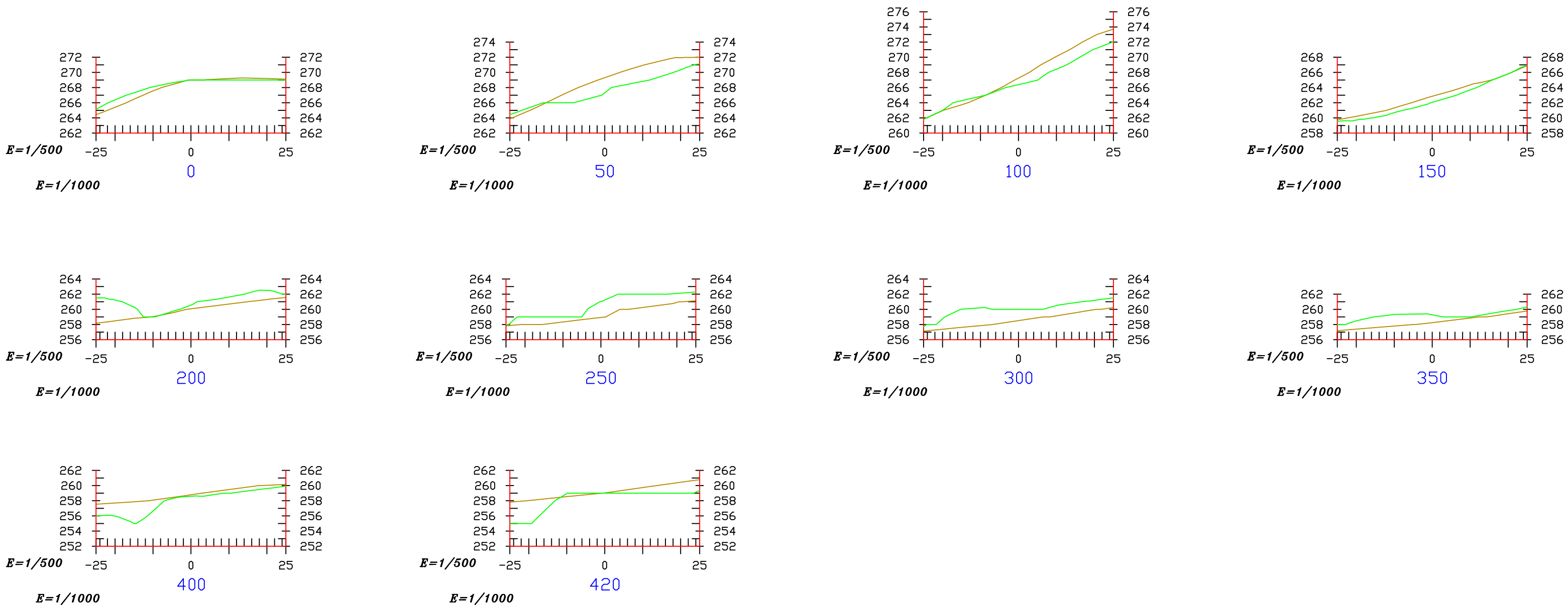
Perfiles Transversales (Secciones cada 50 m)
