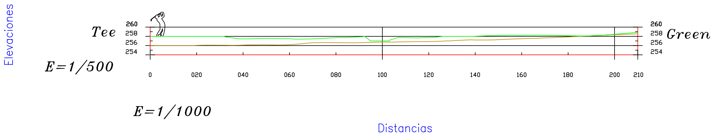
Perfil Longitudinal Hoyo 15
