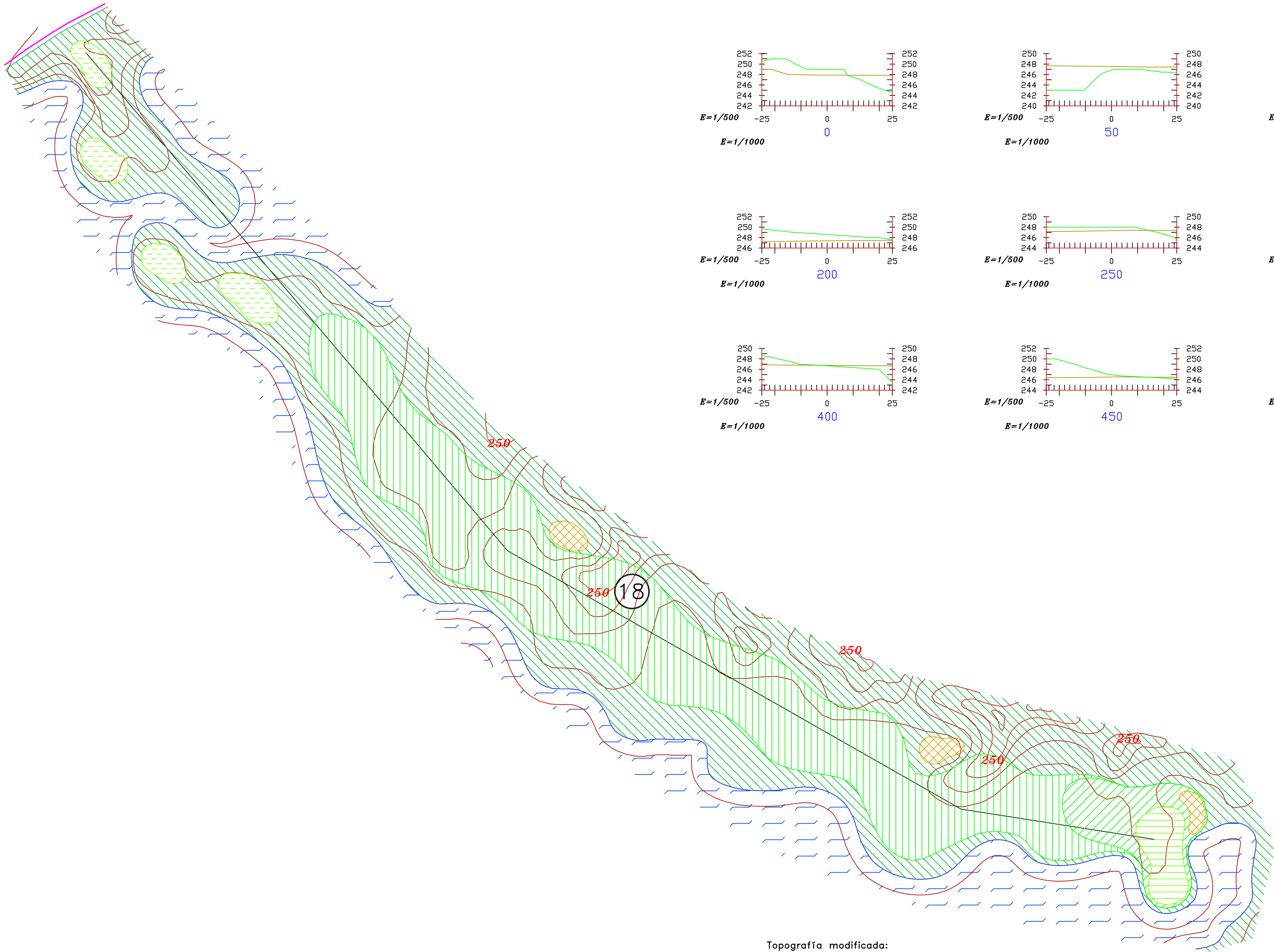
Perfiles Transversales (Secciones cada 50 m)
