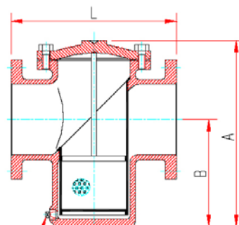
Tapón para tamaños DN 65 a DN 150
