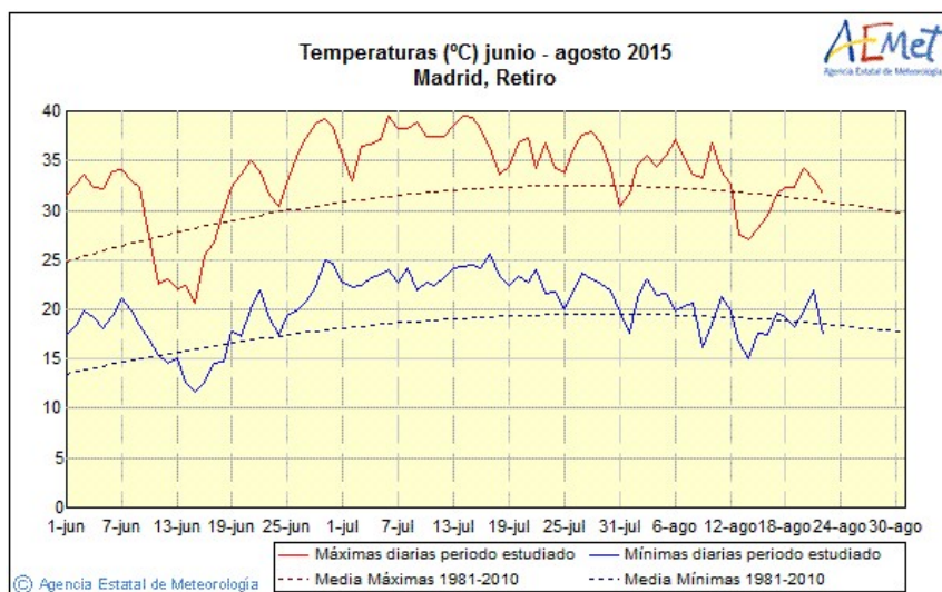
Gráfica 1: Evolución de las temperaturas en Agosto de 2015
