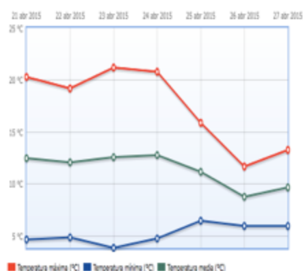
Gráfica 1. Evolución temperaturas durante este mes
